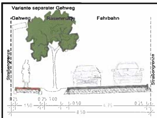
Profil Stückener Straße (Variante)
