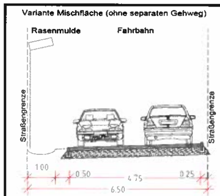
Profil der Wohngebietsstraße
